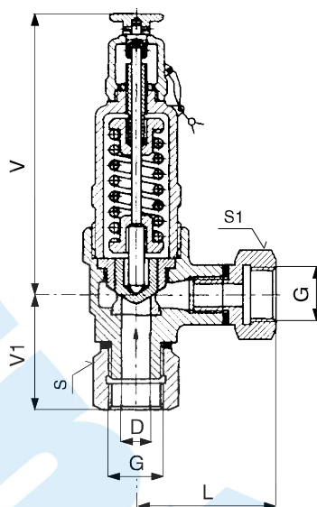
Připojovací a stavební rozměry
