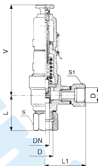
Připojovací a stavební rozměry
